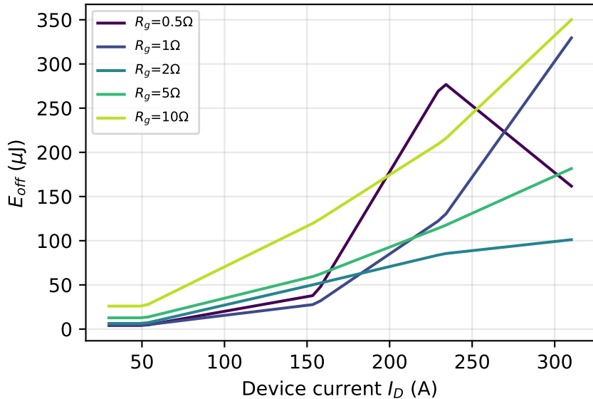
E_{off} vs I_D , L_{loop}=0.7 nH
