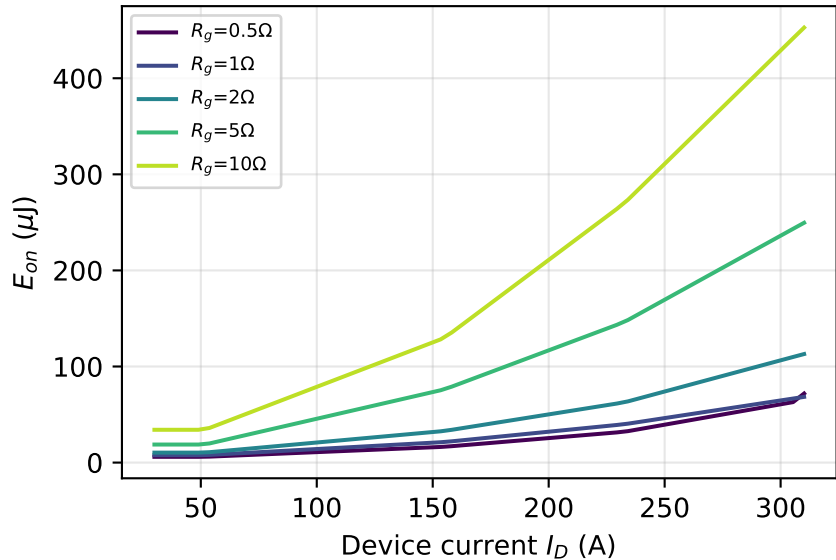
E_{on} vs I_D , L_{loop}=0.7 nH
