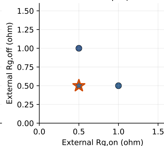
3 nH / 45 A | 9 pairs
