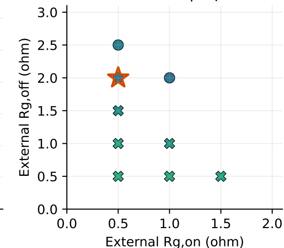
5 nH / 45 A | 576 pairs
