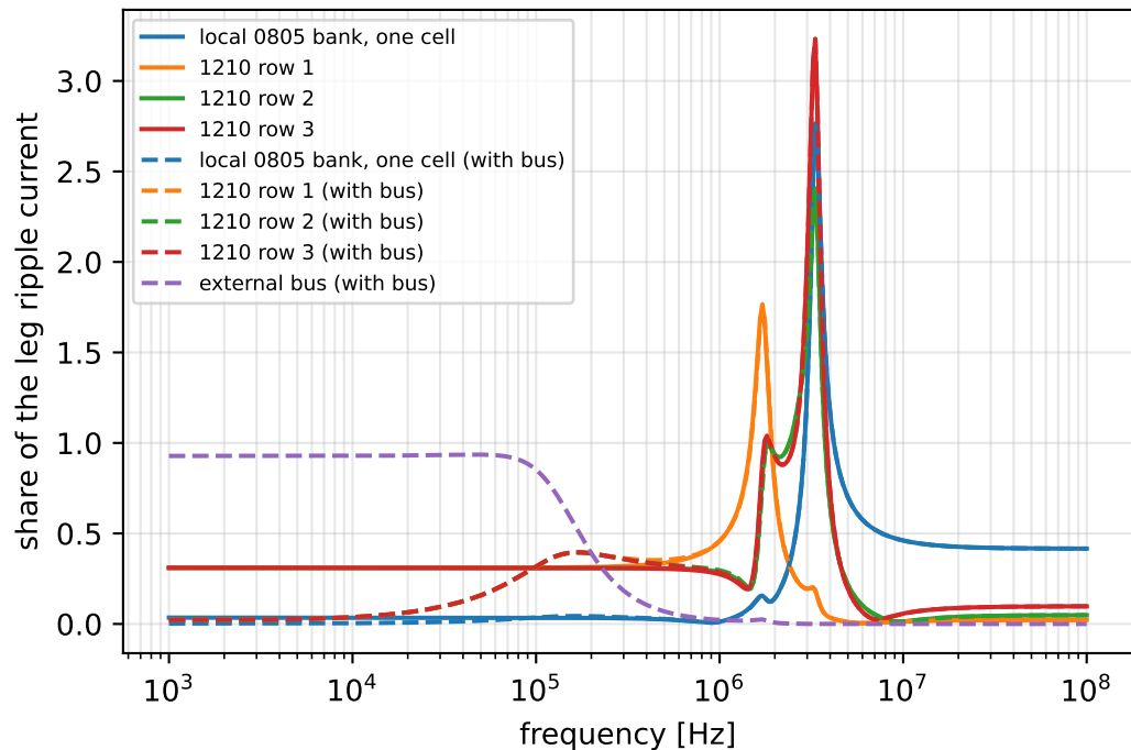
Current division (Q3D copper + capacitor C/ESR/ESL)
