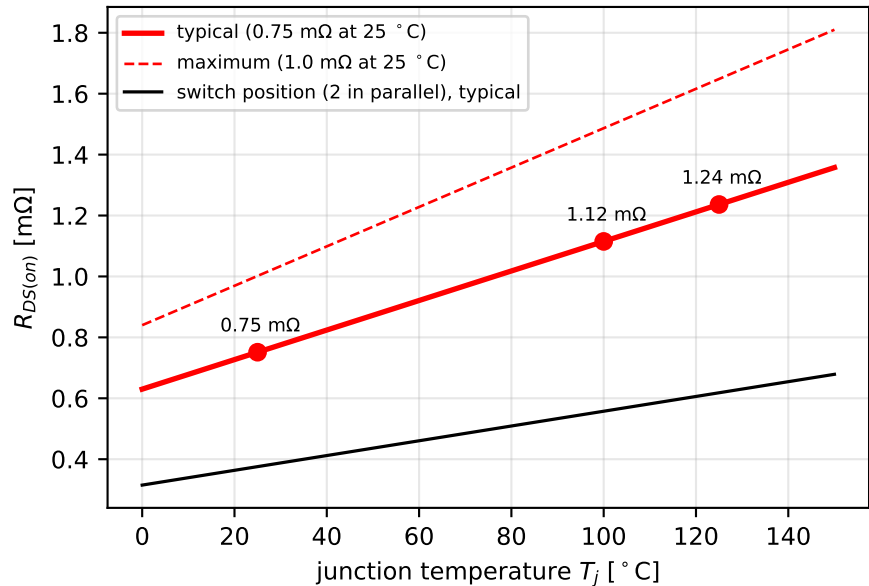
EPC2361 (datasheet Fig. 9, I_D = 50 A, V_{GS} = 5 V)
