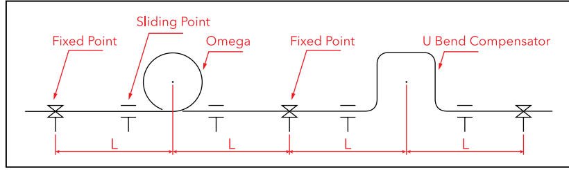
Şekil - 1 Omega ve U parçası
