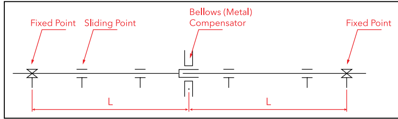
Şekil - 2 Metal kompensatör
