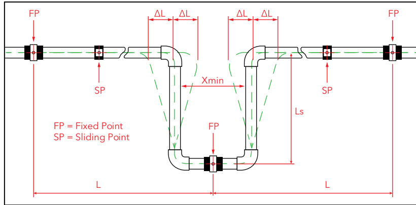
Şekil - 3 U parçası (bükme parçası mesafesinin hesaplanması)
