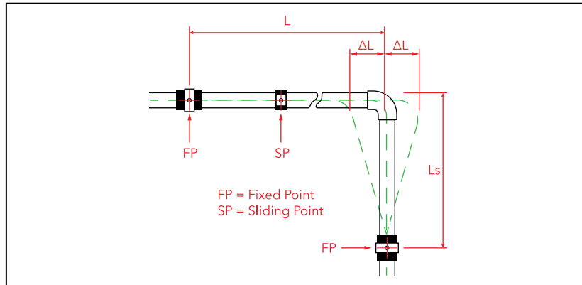
Şekil - 4 Bükme parçası mesafesinin hesaplanması
