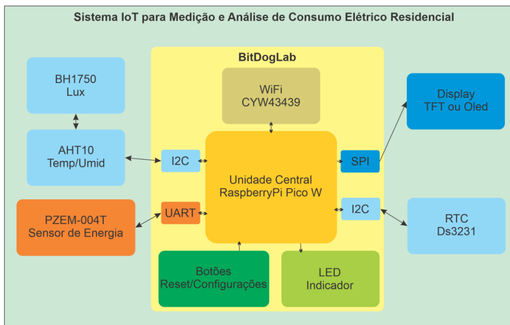
Fig. 5 – Diagrama em blocos – Sujeito a alterações
