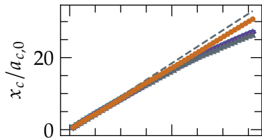
Core trajectory
