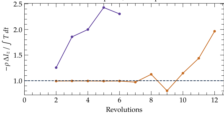
Wake impulse / blade impulse
