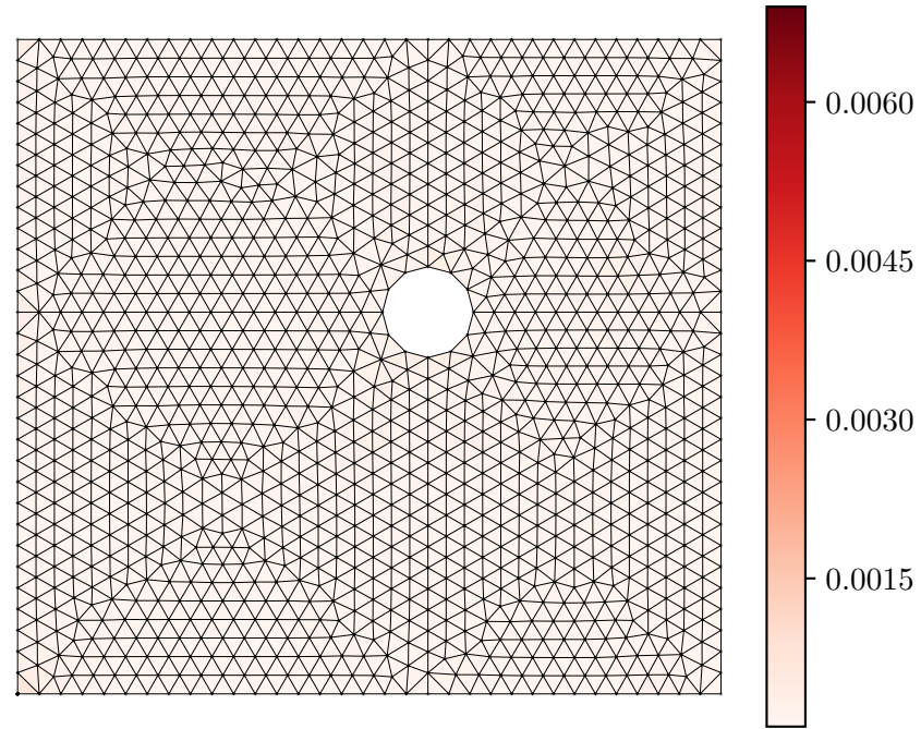
Error |\varepsilon_{xx}^{pred} - \varepsilon_{xx}^{act}|
