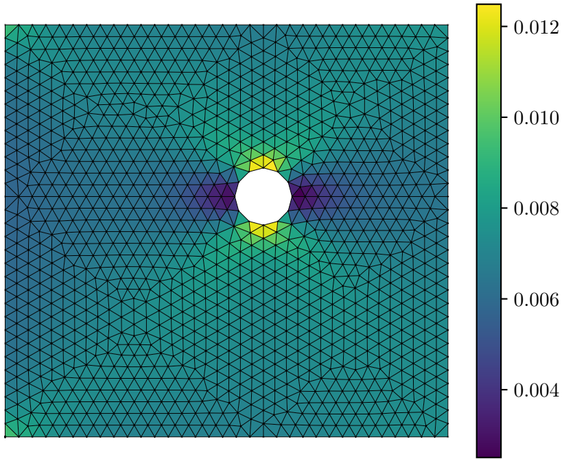
Actual Strain \varepsilon_{xx}
