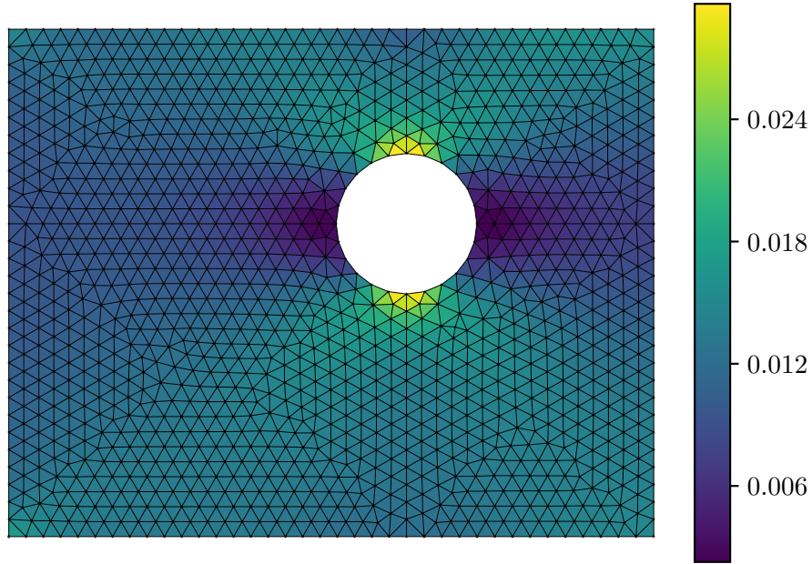
Actual Strain \varepsilon_{xx}
