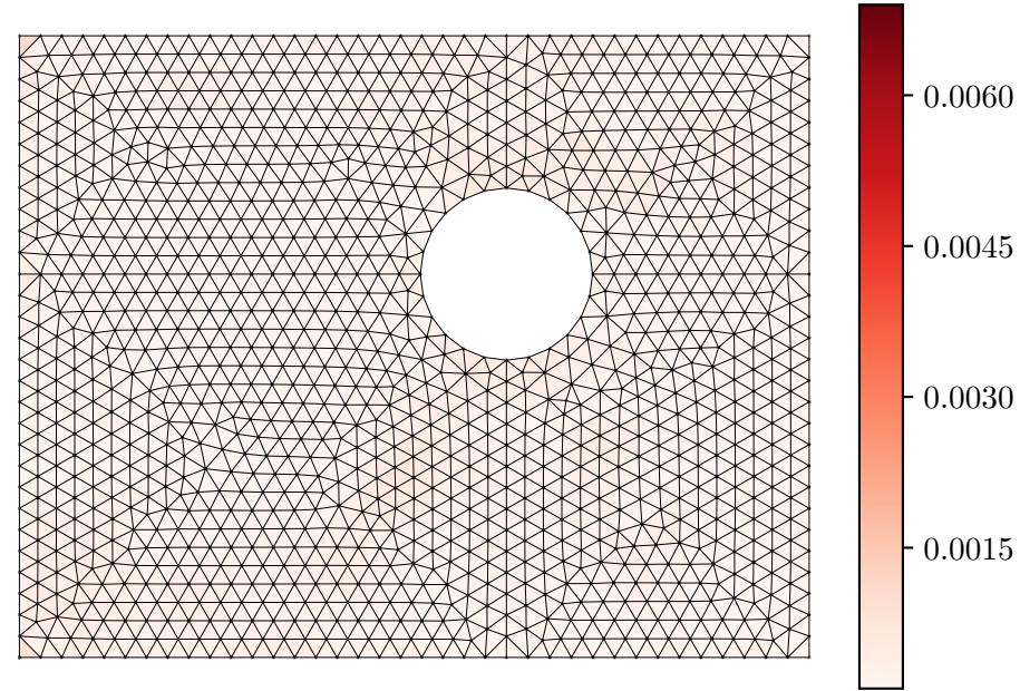
Error |\varepsilon_{xx}^{pred} - \varepsilon_{xx}^{act}|
