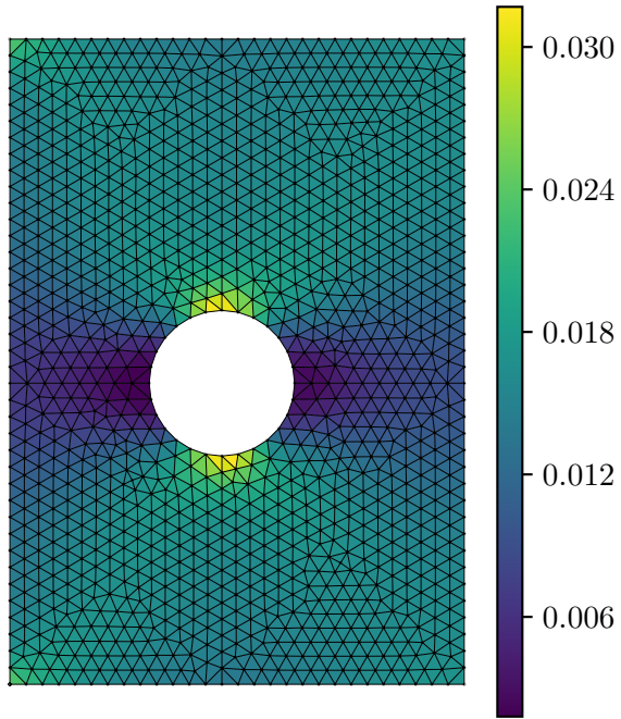
Actual Strain \varepsilon_{xx}
