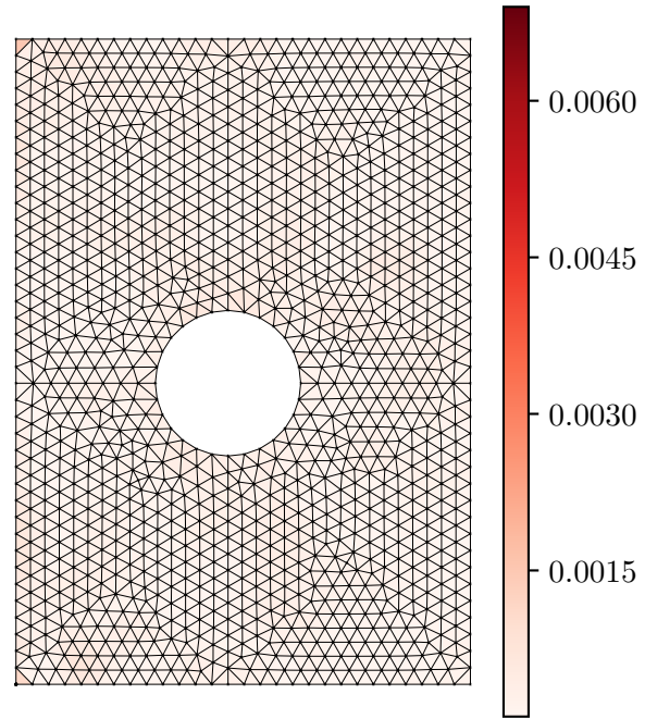
Error |\varepsilon_{xx}^{pred} - \varepsilon_{xx}^{act}|
