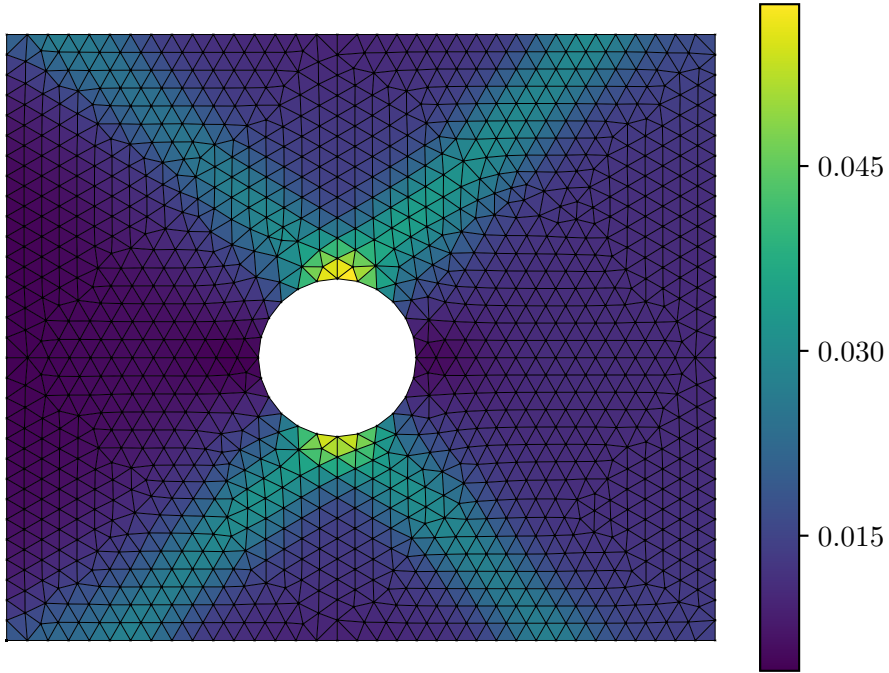
Actual Strain \varepsilon_{xx}
