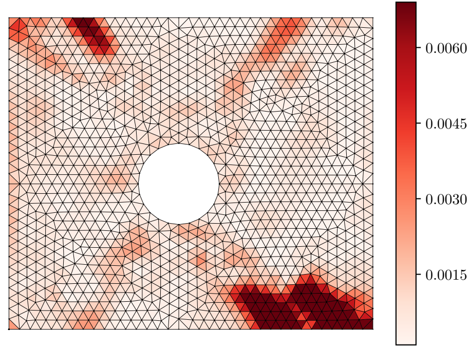
Error |\varepsilon_{xx}^{pred} - \varepsilon_{xx}^{act}|
