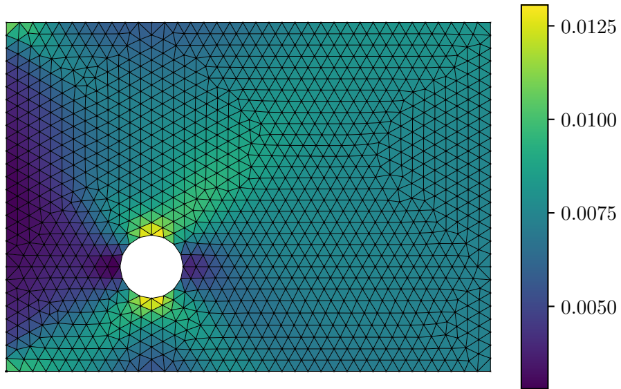
Actual Strain \varepsilon_{xx}
