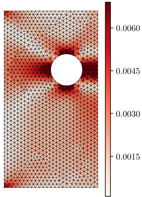
Error |\varepsilon_{xx}^{pred} - \varepsilon_{xx}^{act}|
