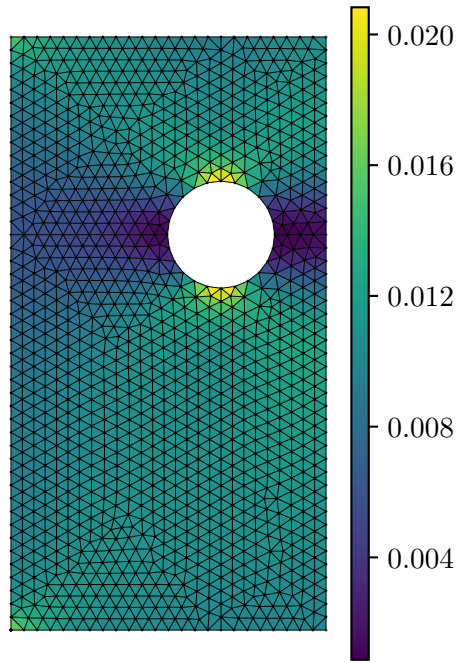
Actual Strain \varepsilon_{xx}
