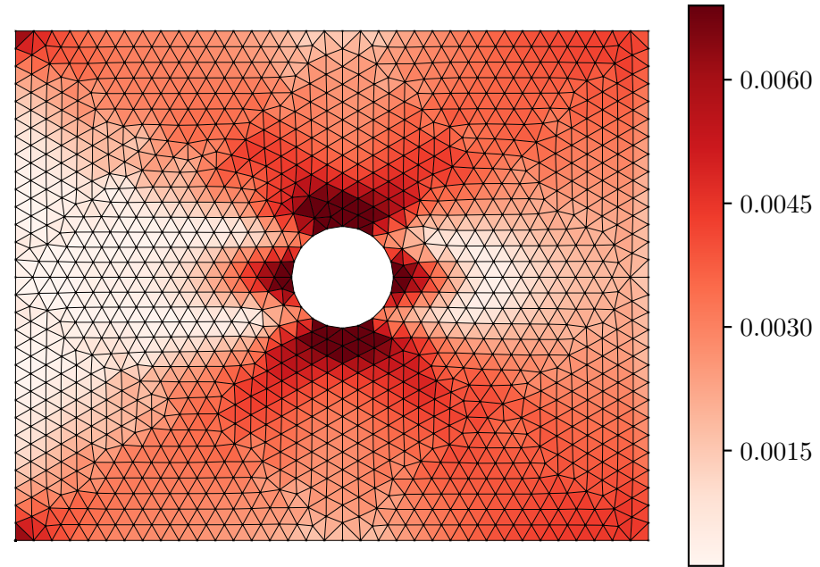
Error |\varepsilon_{xx}^{pred} - \varepsilon_{xx}^{act}|
