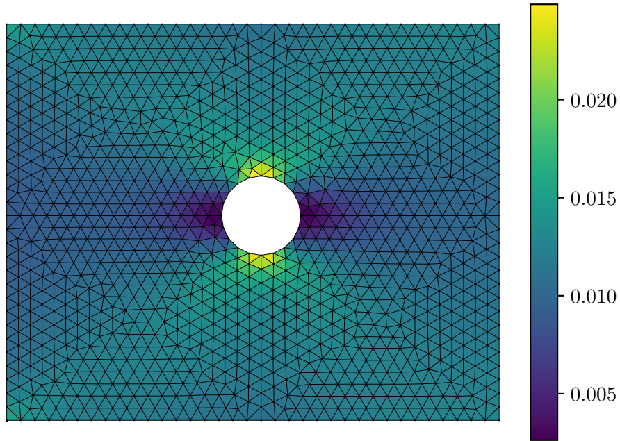
Actual Strain \varepsilon_{xx}
