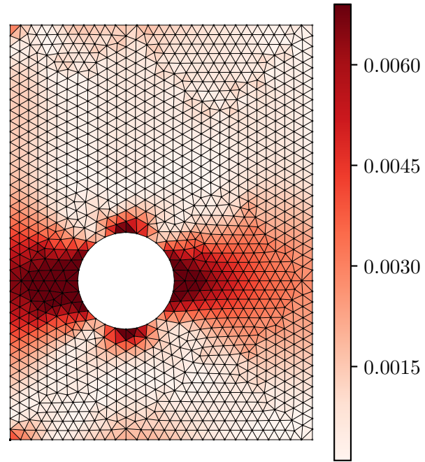
Error |\varepsilon_{xx}^{pred} - \varepsilon_{xx}^{act}|
