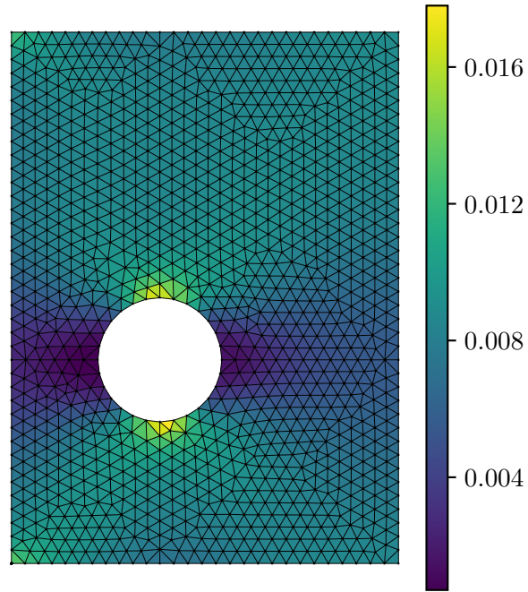
Actual Strain \varepsilon_{xx}
