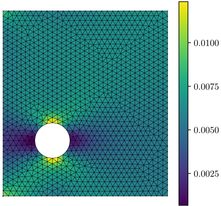
Actual Strain \varepsilon_{xx}
