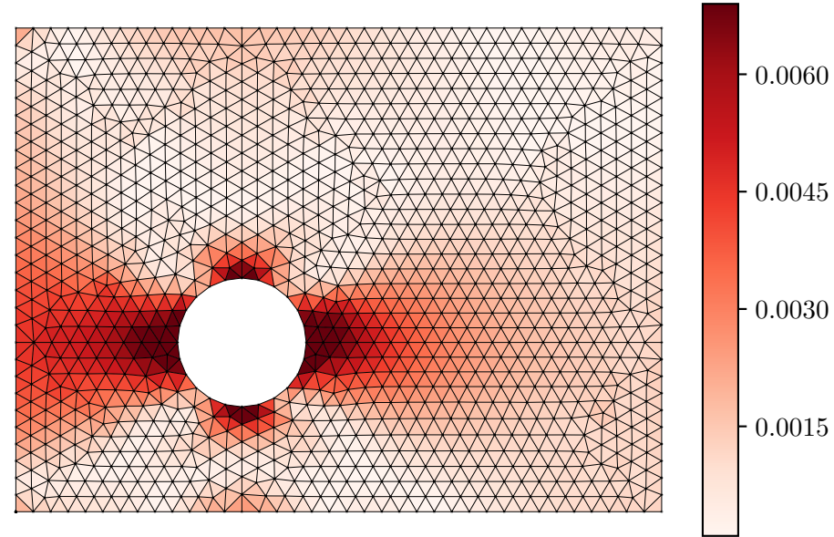
Error |\varepsilon_{xx}^{pred} - \varepsilon_{xx}^{act}|
