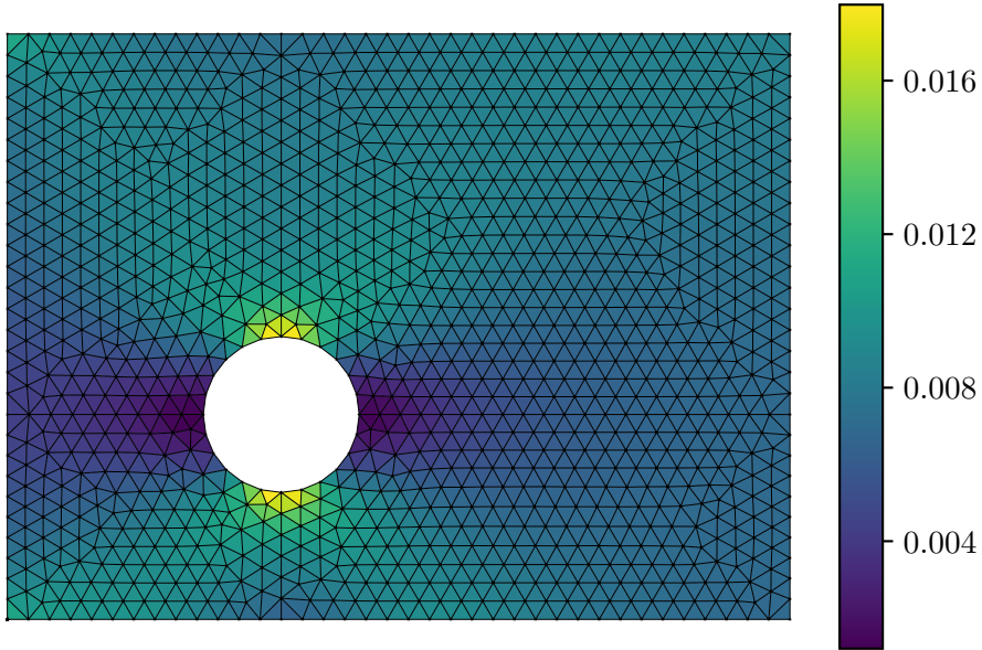
Actual Strain \varepsilon_{xx}
