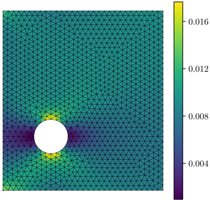
Actual Strain \varepsilon_{xx}
