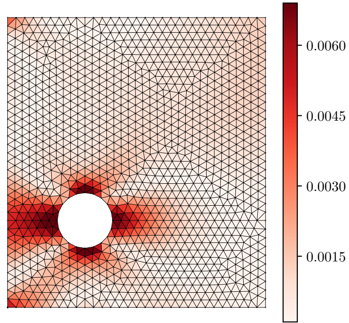
Error |\varepsilon_{xx}^{pred} - \varepsilon_{xx}^{act}|
