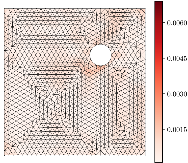
Error |\varepsilon_{xx}^{pred} - \varepsilon_{xx}^{act}|
