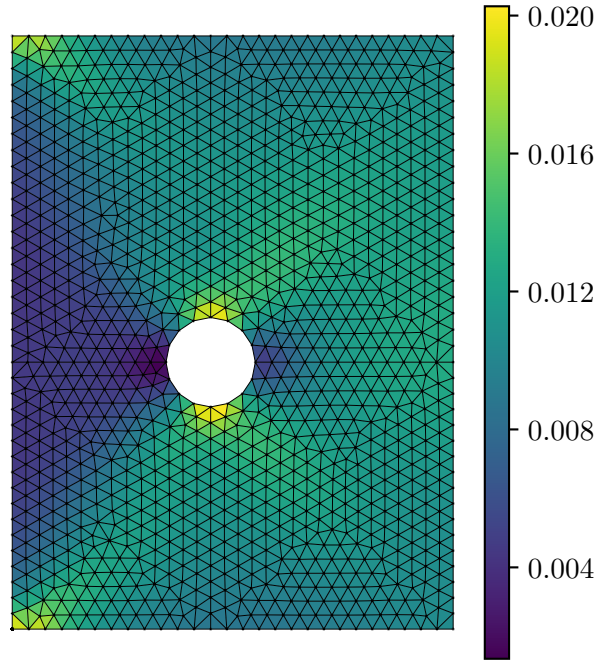
Actual Strain \varepsilon_{xx}
