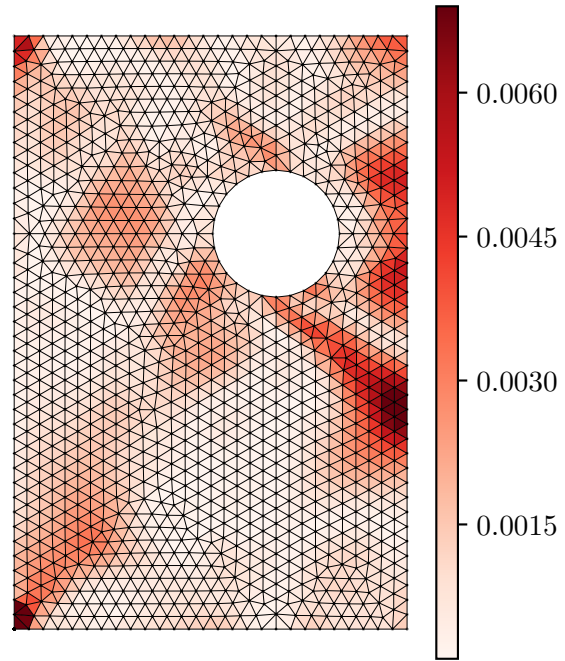
Nominal Error |\varepsilon_{xx}^{pred} - \varepsilon_{xx}^{act}|
