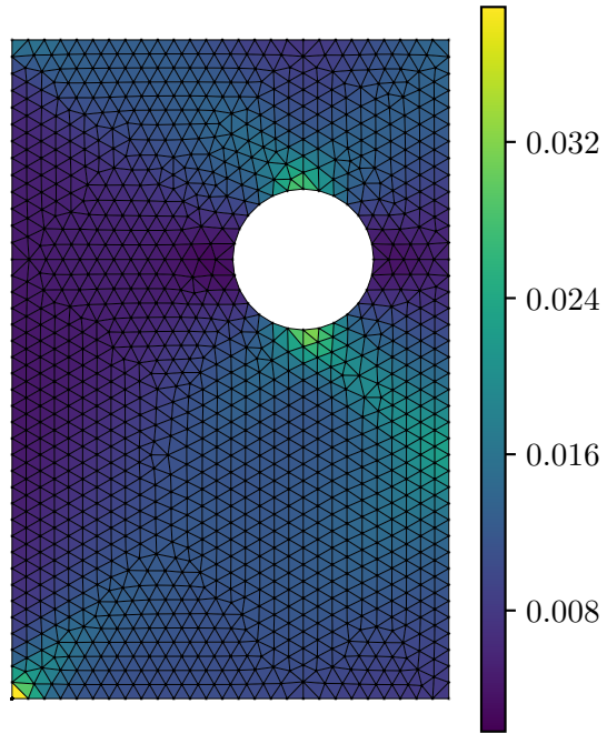
Actual Strain \varepsilon_{xx}
