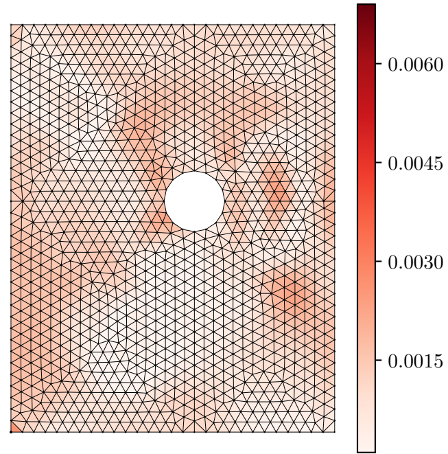
Nominal Error |\varepsilon_{xx}^{pred} - \varepsilon_{xx}^{act}|
