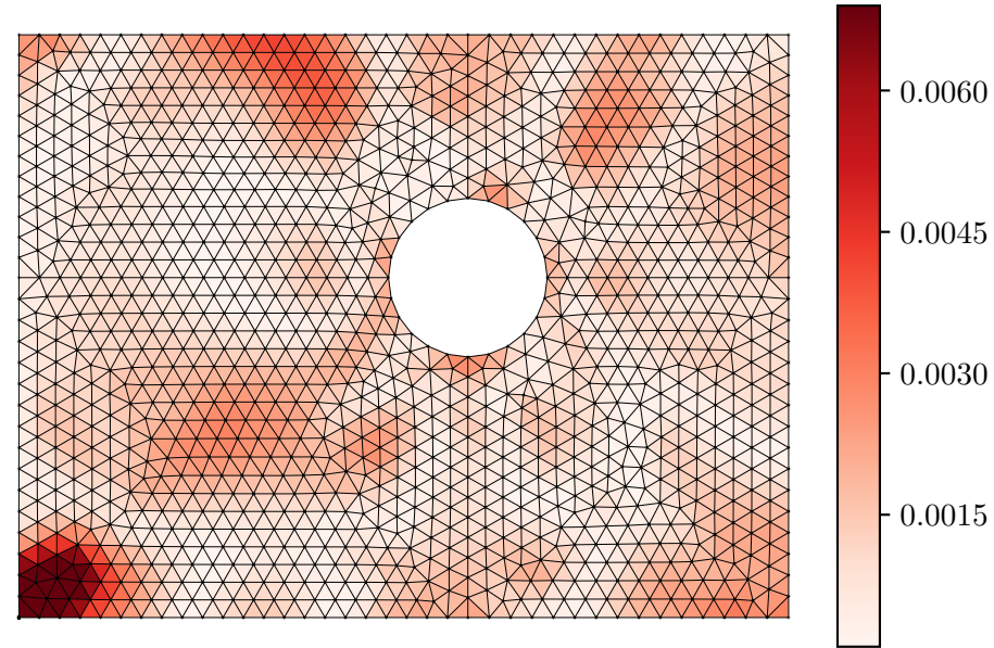
Nominal Error |\varepsilon_{xx}^{pred} - \varepsilon_{xx}^{act}|
