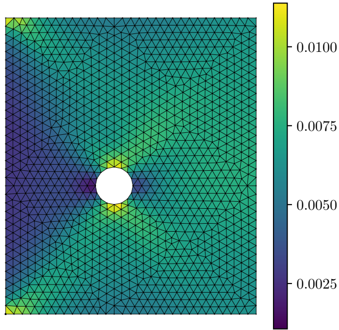
Actual Strain \varepsilon_{xx}
