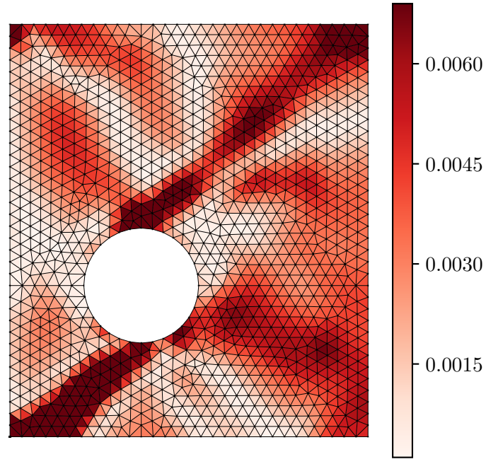
Nominal Error |\varepsilon_{xx}^{pred} - \varepsilon_{xx}^{act}|
