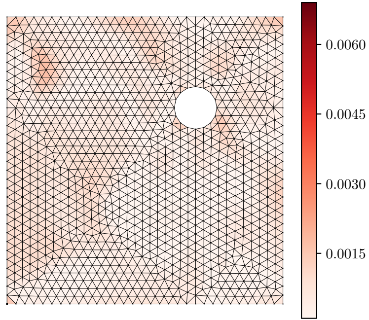
Nominal Error |\varepsilon_{xx}^{pred} - \varepsilon_{xx}^{act}|
