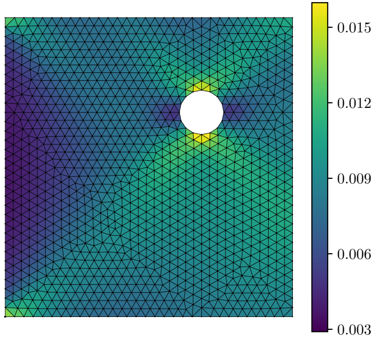
Actual Strain \varepsilon_{xx}
