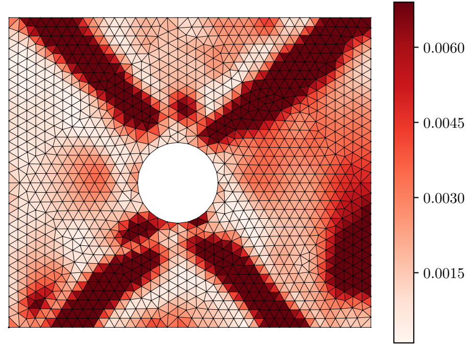
Nominal Error |\varepsilon_{xx}^{pred} - \varepsilon_{xx}^{act}|
