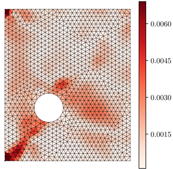
Nominal Error |\varepsilon_{xx}^{pred} - \varepsilon_{xx}^{act}|
