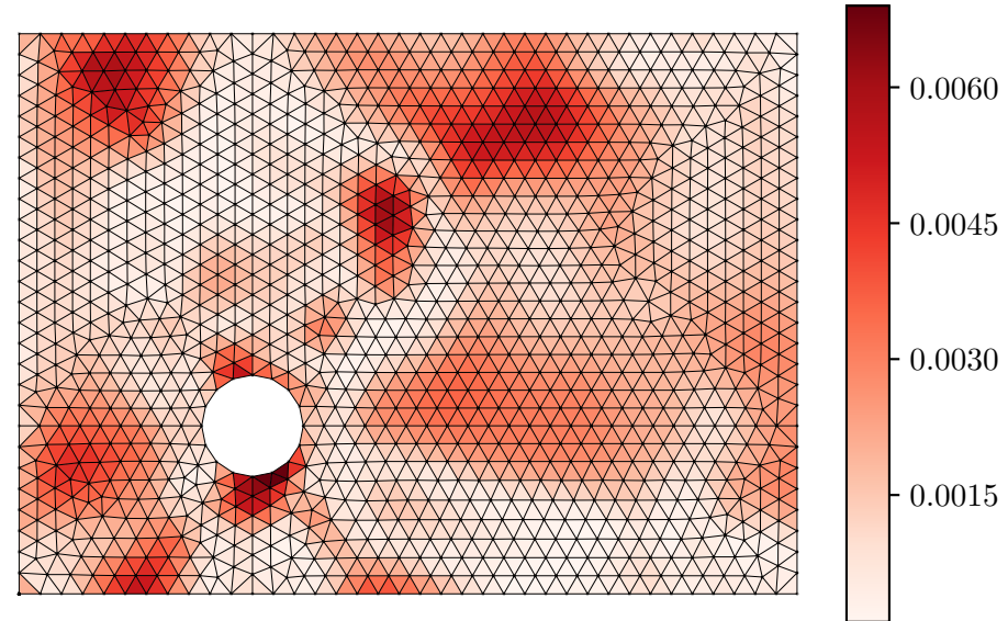
Nominal Error |\varepsilon_{xx}^{pred} - \varepsilon_{xx}^{act}|
