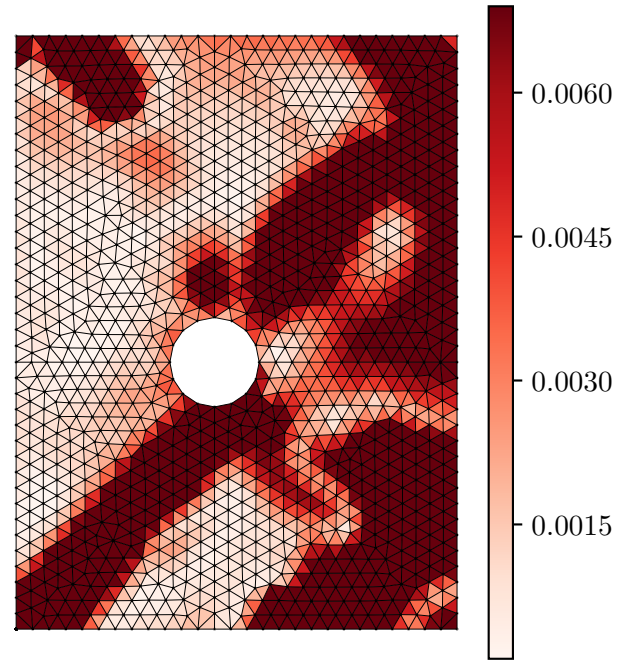
Nominal Error |\varepsilon_{xx}^{pred} - \varepsilon_{xx}^{act}|
