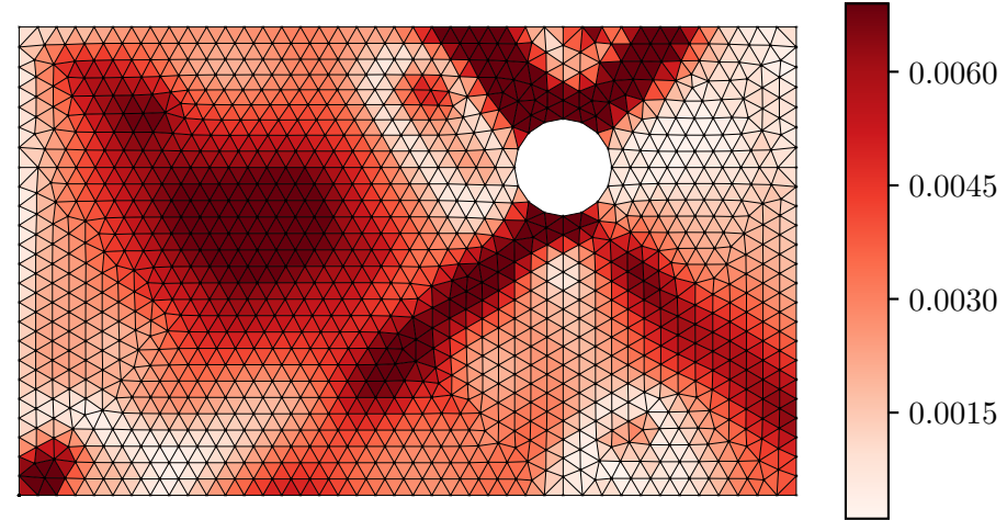
Nominal Error |\varepsilon_{xx}^{pred} - \varepsilon_{xx}^{act}|
