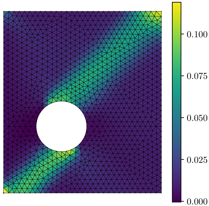
Actual Strain \varepsilon_{xx}
