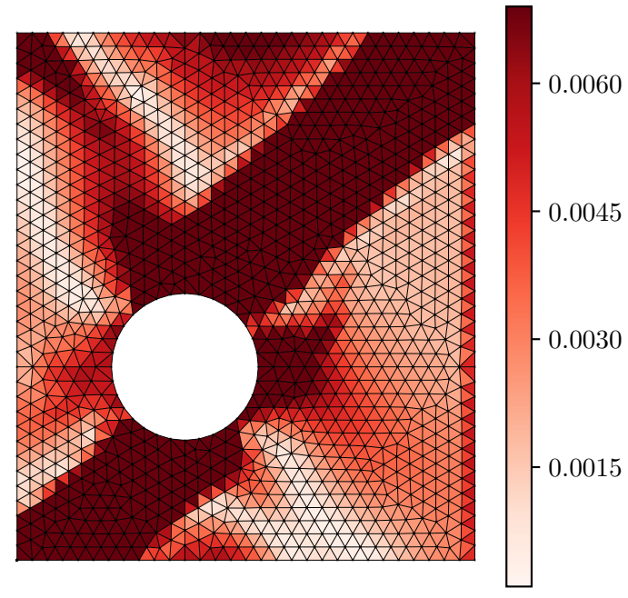
Error |\varepsilon_{xx}^{pred} - \varepsilon_{xx}^{act}|
