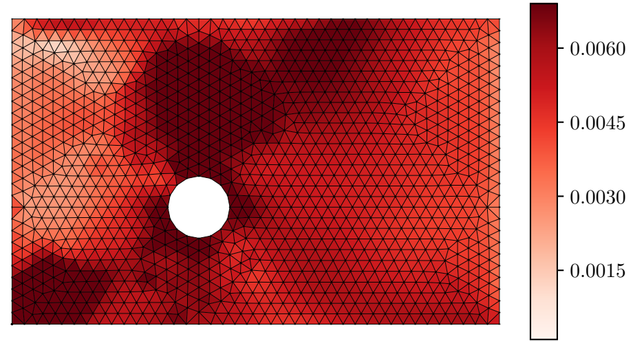
Error |\varepsilon_{xx}^{pred} - \varepsilon_{xx}^{act}|
