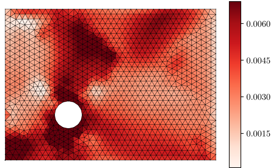
Error |\varepsilon_{xx}^{pred} - \varepsilon_{xx}^{act}|
