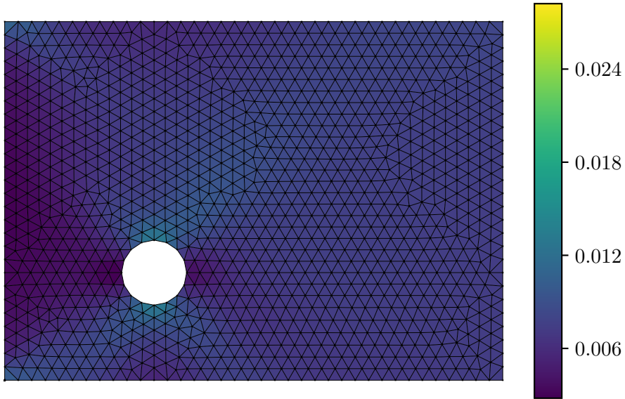
Actual Strain \varepsilon_{xx}
