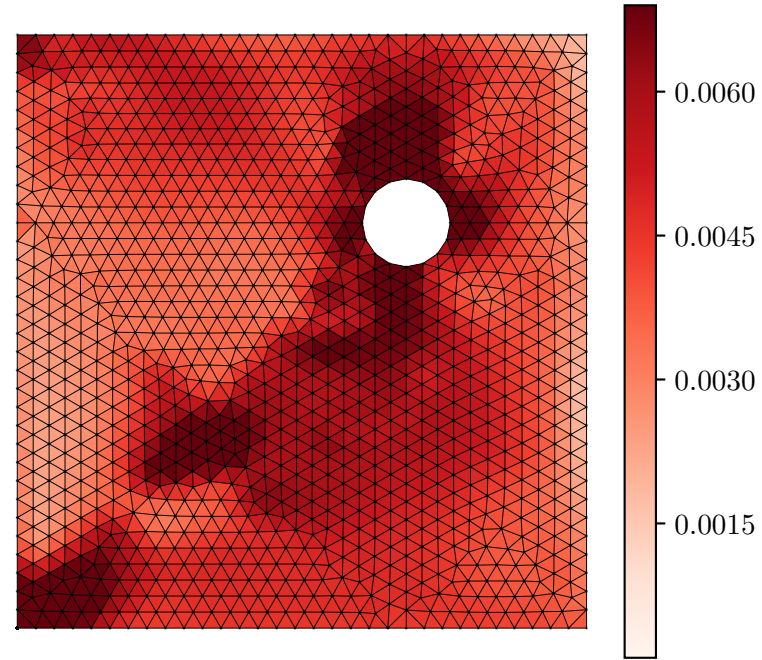
Error |\varepsilon_{xx}^{pred} - \varepsilon_{xx}^{act}|
