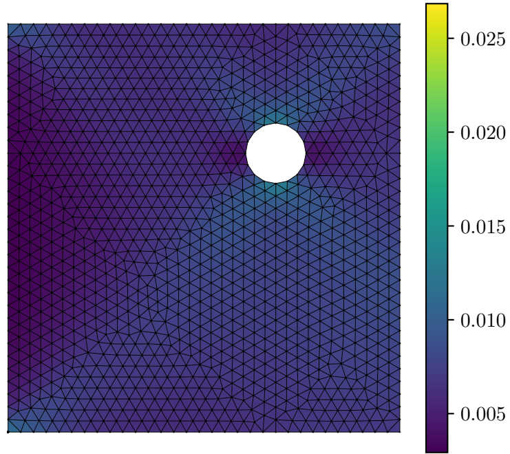
Actual Strain \varepsilon_{xx}
