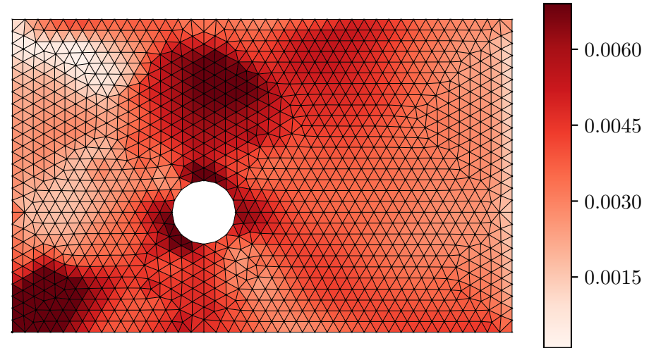
Error |\varepsilon_{xx}^{pred} - \varepsilon_{xx}^{act}|
