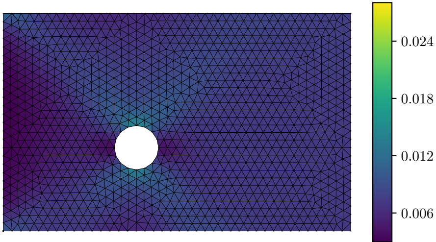
Actual Strain \varepsilon_{xx}
