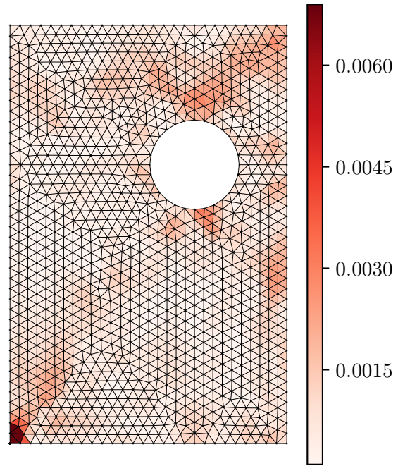
Error |\varepsilon_{xx}^{pred} - \varepsilon_{xx}^{act}|
