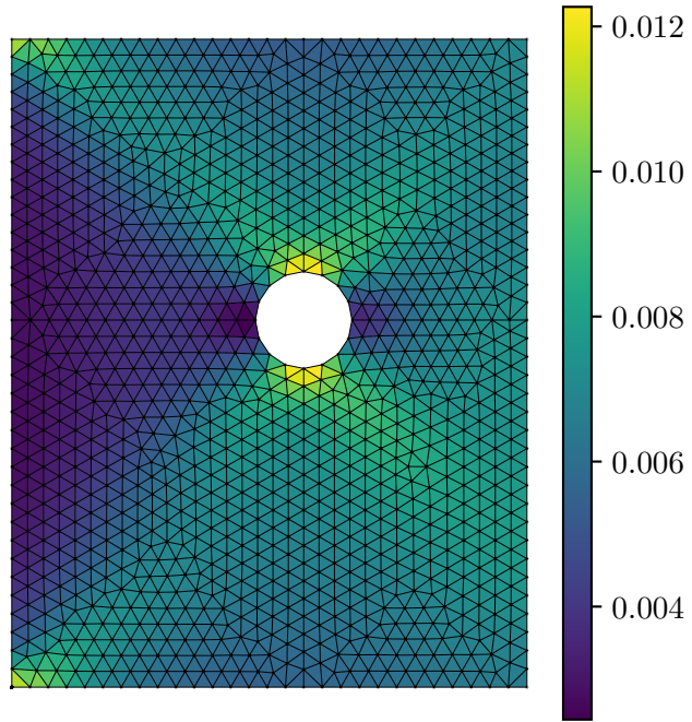
Actual Strain \varepsilon_{xx}
