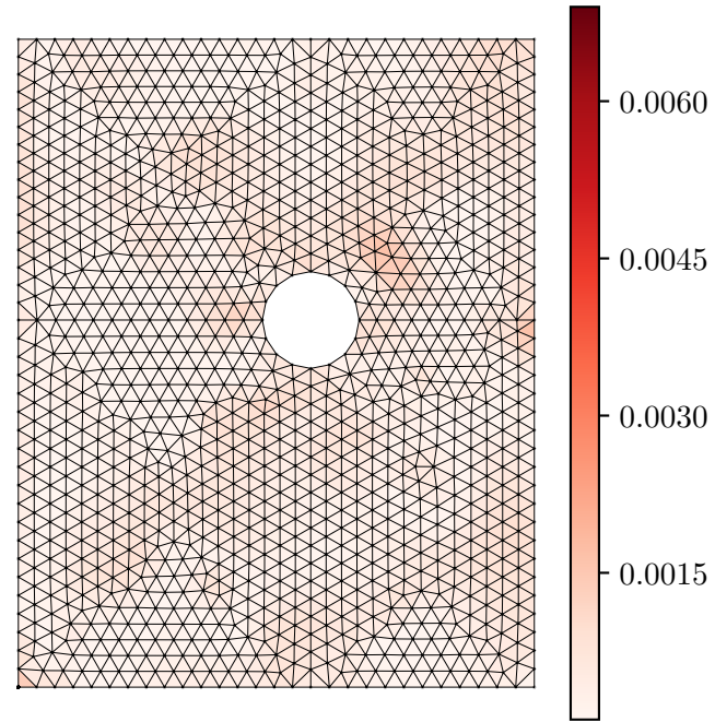
Error |\varepsilon_{xx}^{pred} - \varepsilon_{xx}^{act}|
