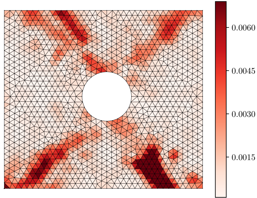
Error |\varepsilon_{xx}^{pred} - \varepsilon_{xx}^{act}|
