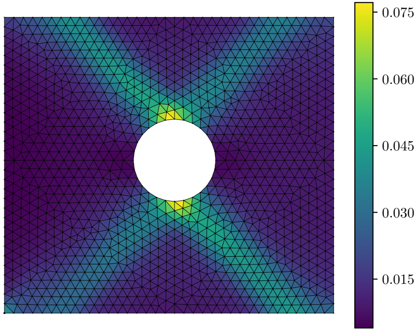
Actual Strain \varepsilon_{xx}
