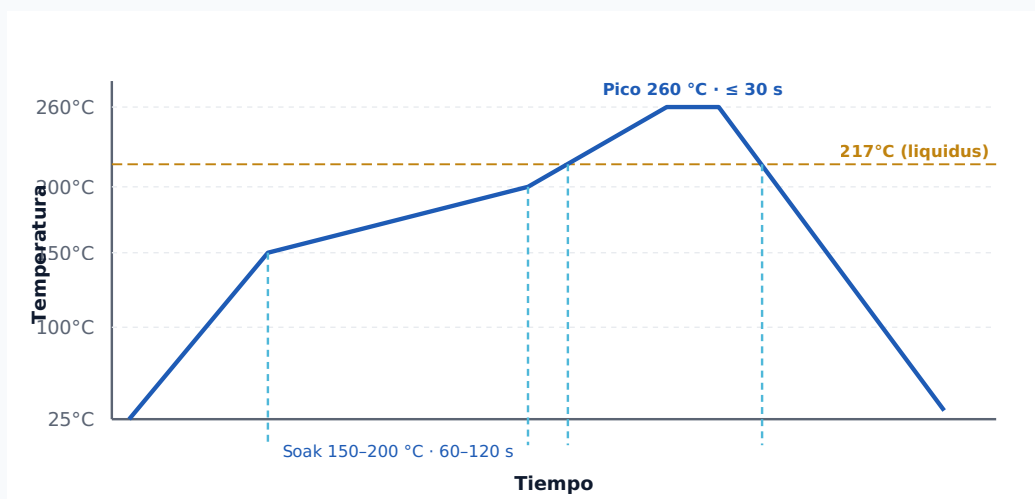
Figura 13: Perfil de temperatura recomendado para reflujo
