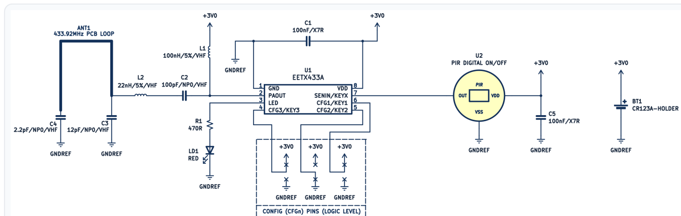
Figura 1: Variante 1 PIR — pirosensor digital único accionando el EETX433A
