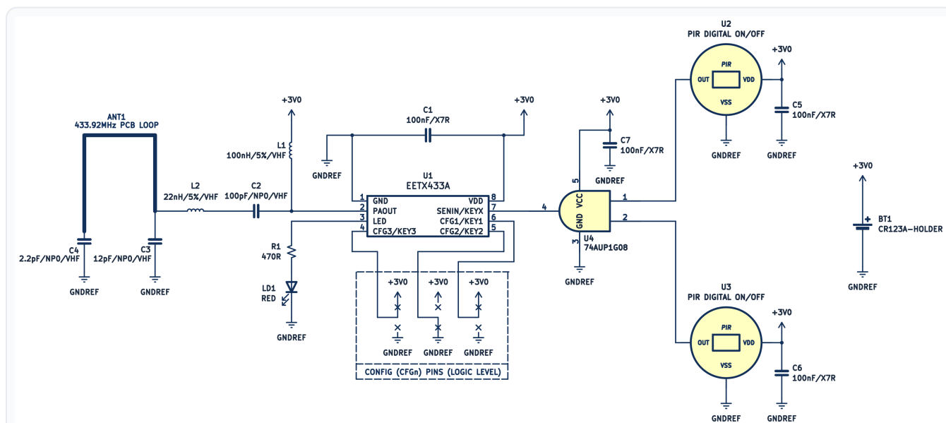
Figura 2: Variante 2 PIR — dos piro sensores + puerta lógica Y (disparo por coincidencia) + EETX433A
