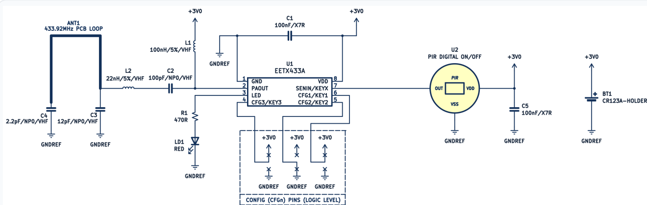
图 7：运动传感器典型应用 (数字 ON/OFF PIR + EETX433A)
