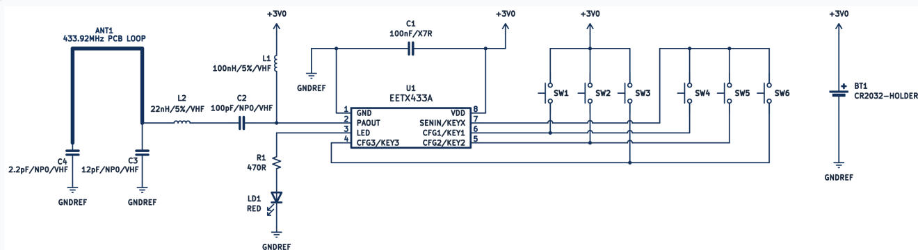
图 5：433.92 MHz 典型应用 — 6 按键
