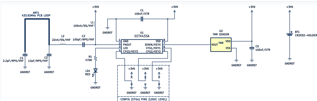
图 6：磁性开关传感器典型应用 (TMR + EETX433A)
