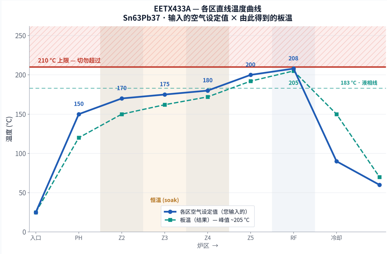
各区曲线 — 空气设定值 × 板温（峰值 ~205 °C · TAL ~64 s · ≤ 210 °C）。
