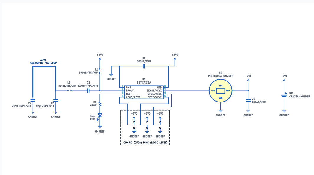
Figura 1: Variante 1 PIR — pirosensor digital único acionando o EETX433A
