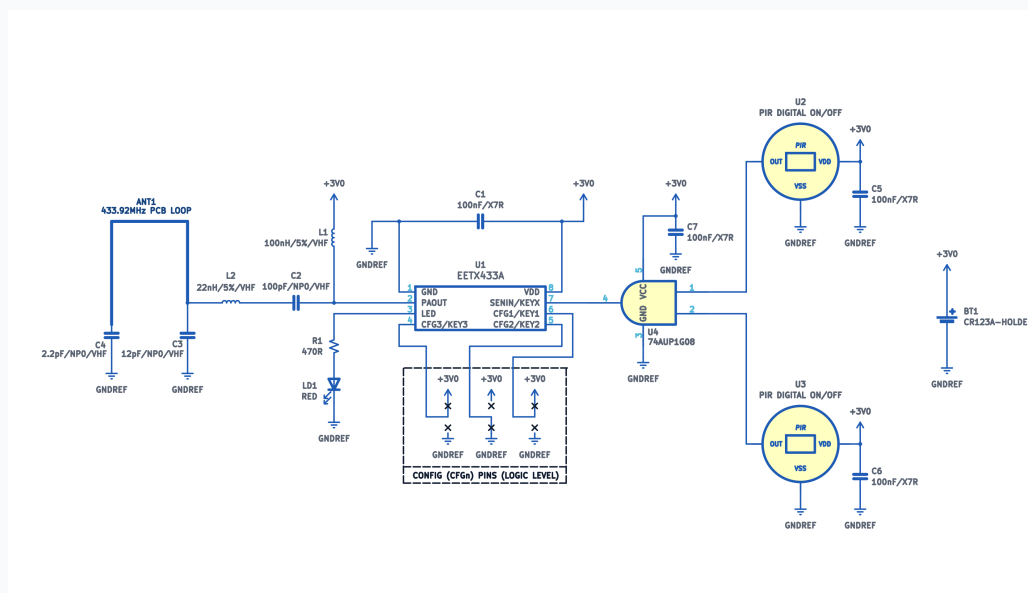
图 2: 2 PIR 方案 — 两个热释电传感器 + 与门（符合触发）+ EETX433A
