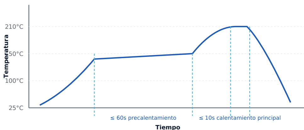
Figura 10: Perfil de temperatura recomendado para reflujo
