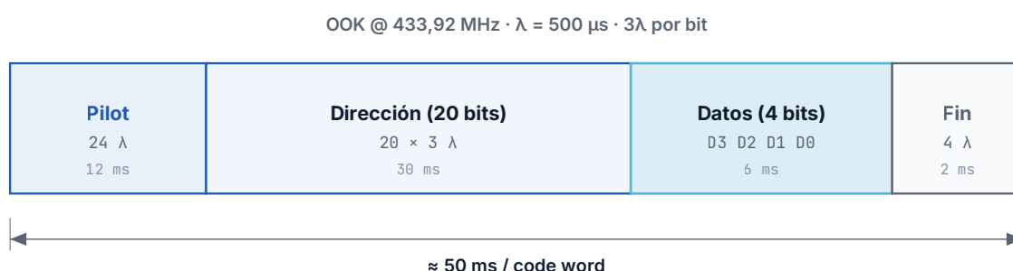
Figura 9: Estructura del paquete de transmisión
