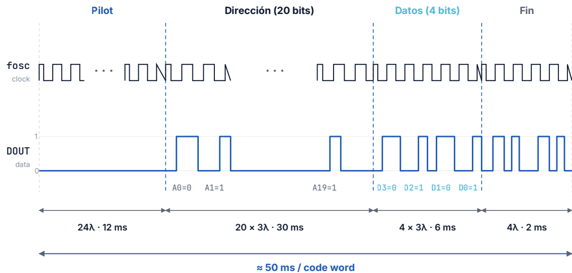
Figura 9b: Cronograma del frame — fosc + DOUT (Pilot · Dirección · Datos · Fin)
