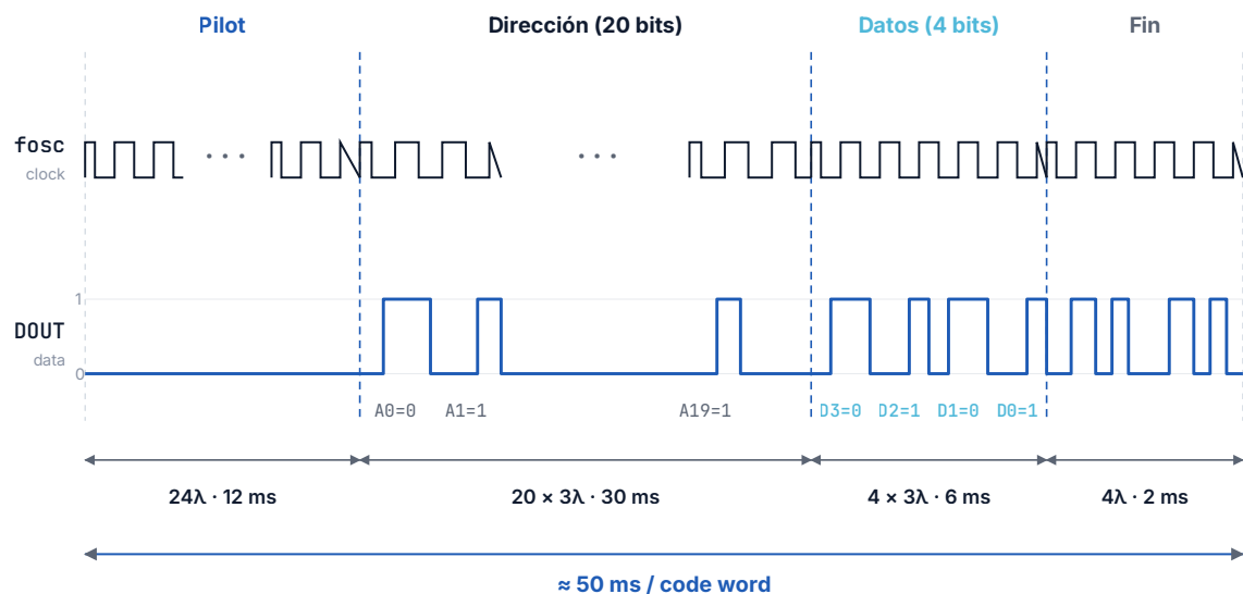
Figura 11: Cronograma del frame — f_{osc} + DOUT (Pilot · Dirección · Datos · Fin)
