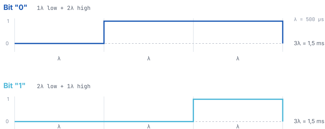
Figura 12: Formas de onda dos bits lógicos (modulação OOK)
