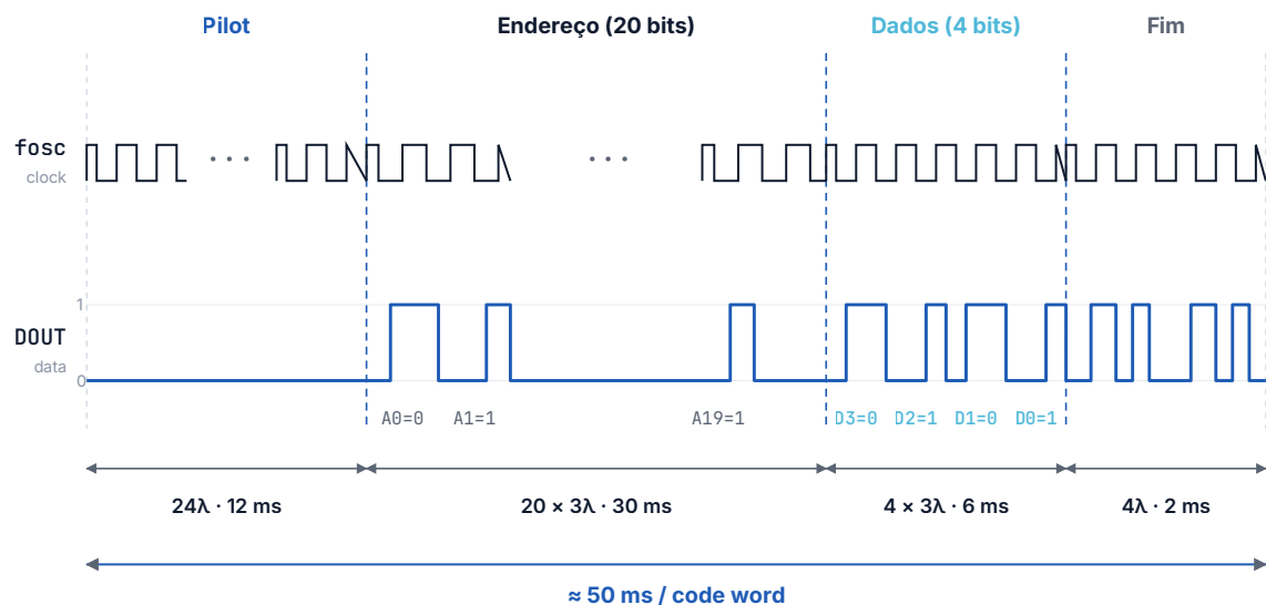
Figura 11: Cronograma do frame — f_{osc} + DOUT (Pilot · Endereço · Dados · Fim)
