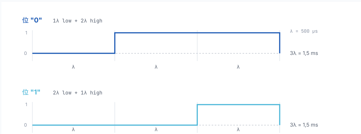
图 10: 逻辑位波形 (OOK 调制)
