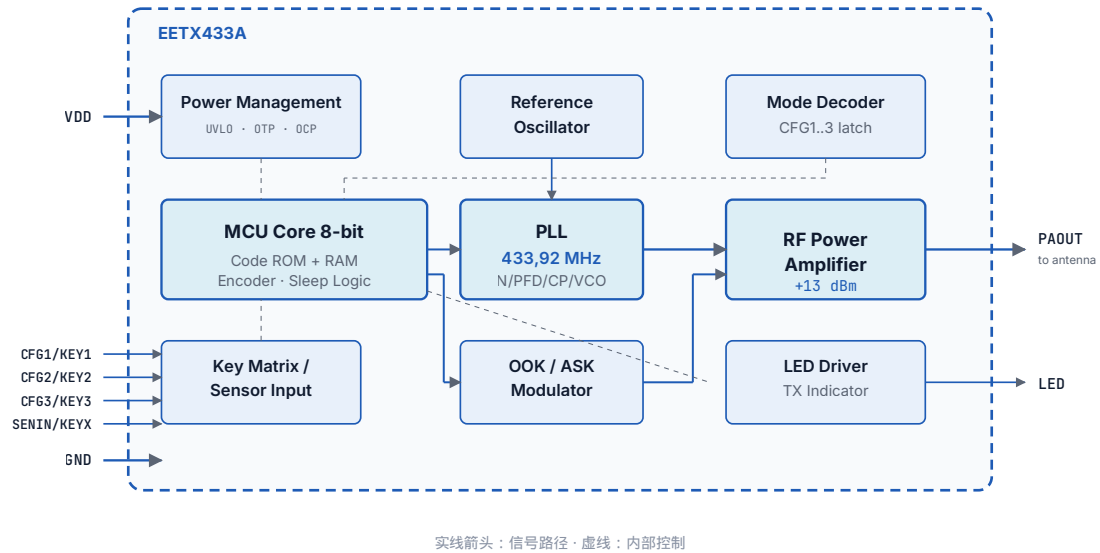
图 0: EETX433A 内部功能框图
