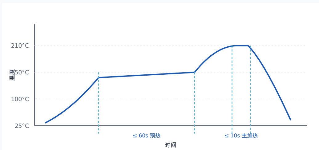
图 11：推荐回流炉温度曲线
