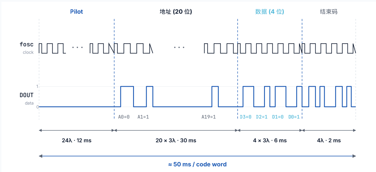
图 9b: 帧时序 — f_{osc} + DOUT (前导码 · 地址 · 数据 · 结束码)
