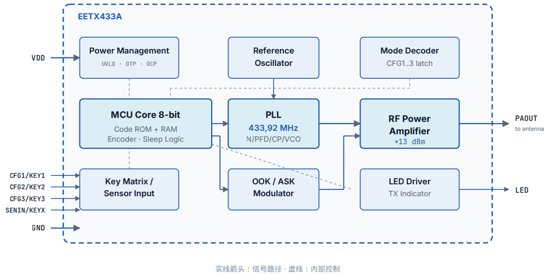
图 1: EETX433A 内部功能框图
