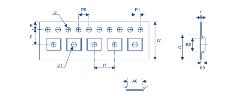
图 16: 12 mm 编带
